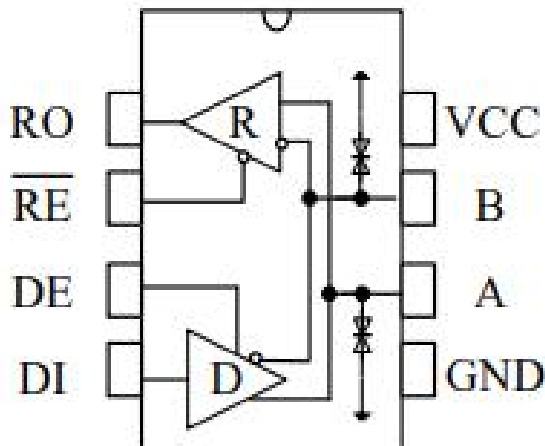
图 1 SN65HVD3082EDR 引脚分布图
