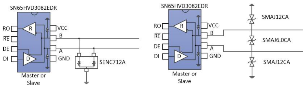
图 11 端口防护方案
