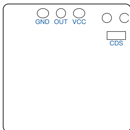
EDC18E 引脚定义
