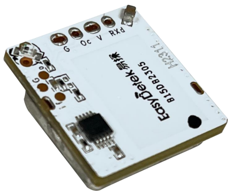
(天线面) EDC15E
