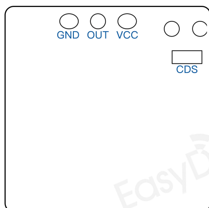
EDC18D 引脚定义
