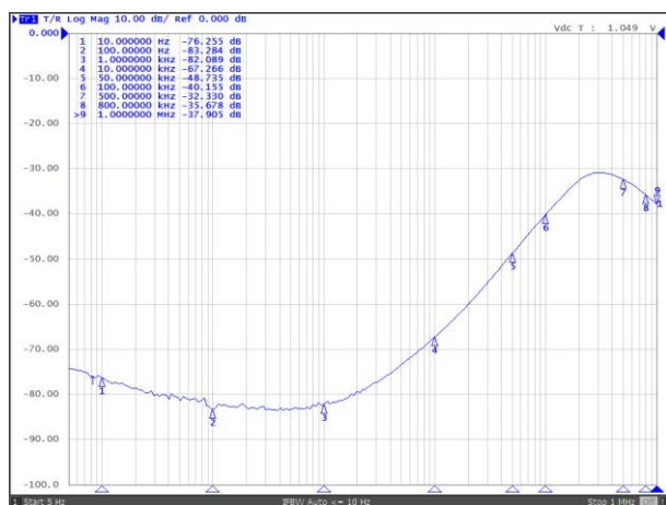
PSRR
