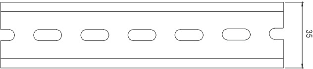
安装导轨:TS35/7.5 或者 TS35/15
