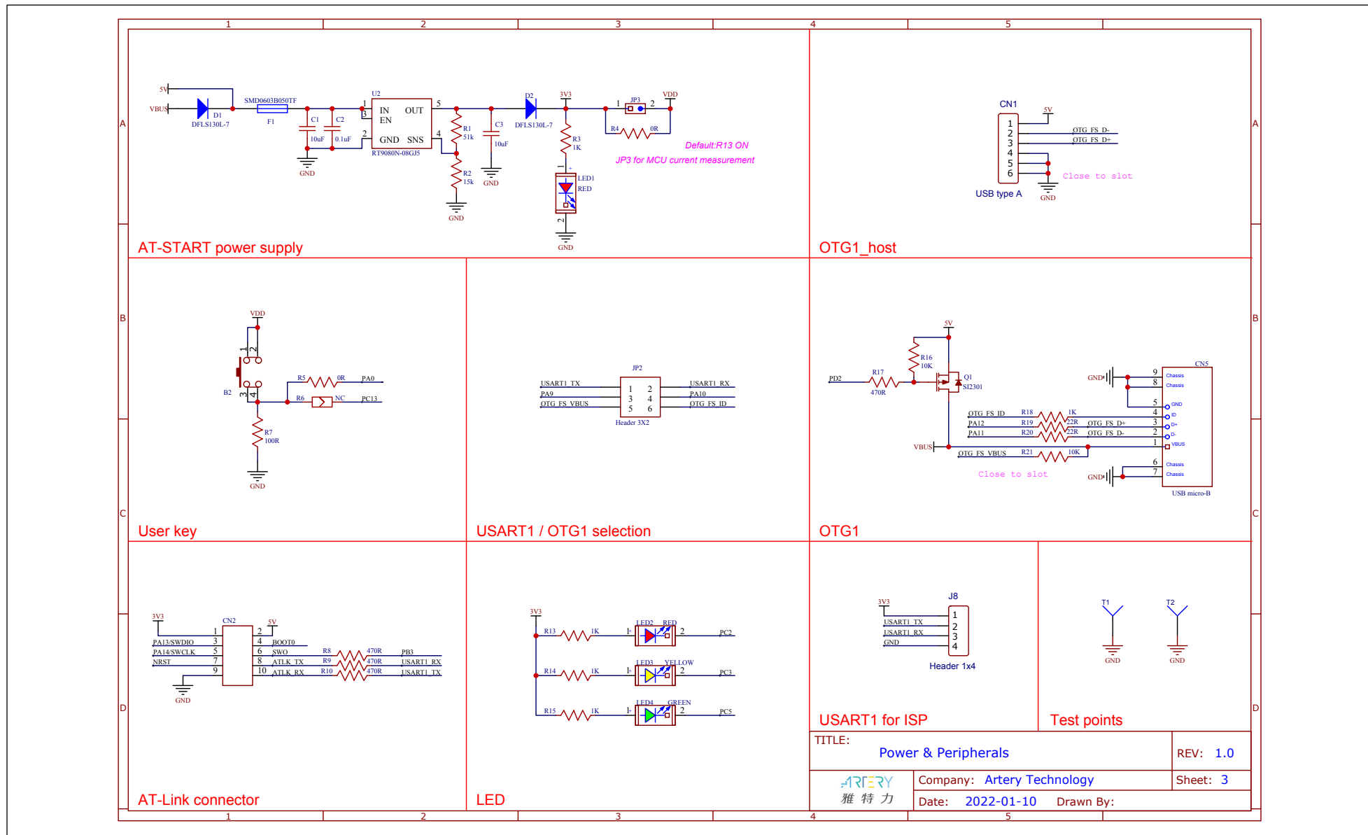
图 6. 原理图 (电源和外设)
