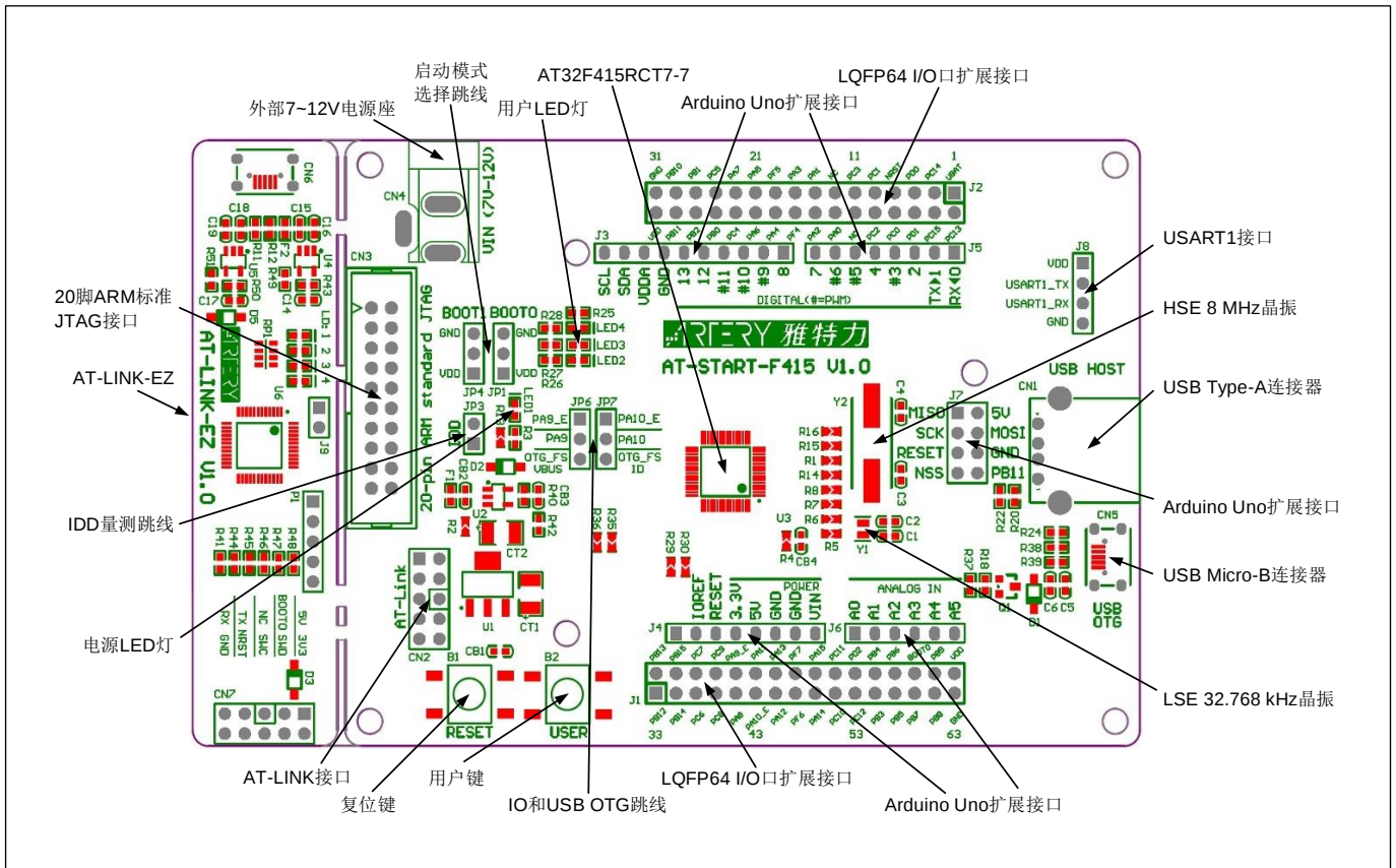
图 3. 顶层布局
