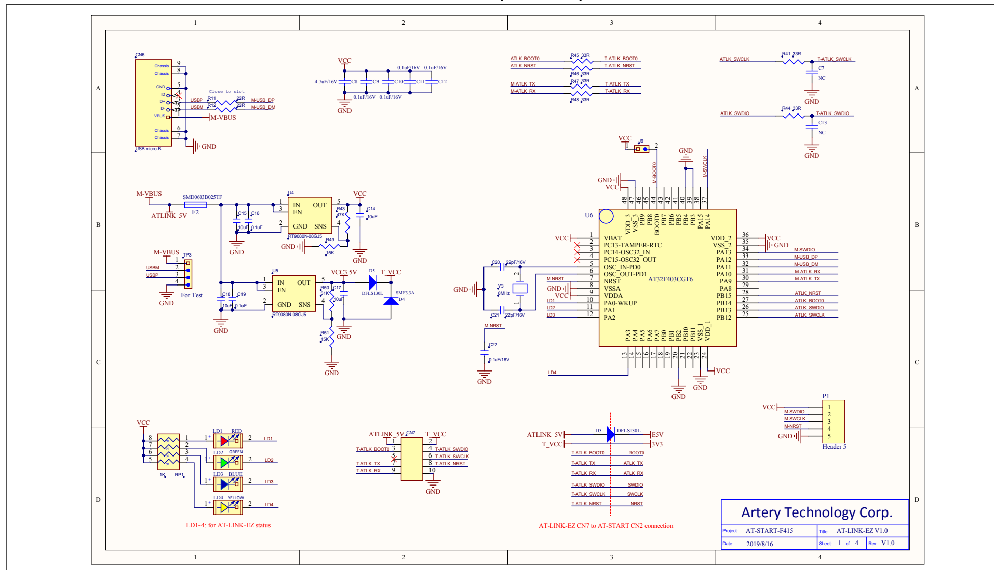
图 6. 原理图(AT-LINK-EZ)
