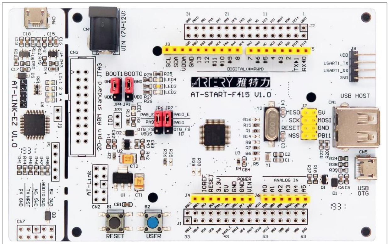
图 1. AT-START-F415 及 AT-LINK-EZ 外观
