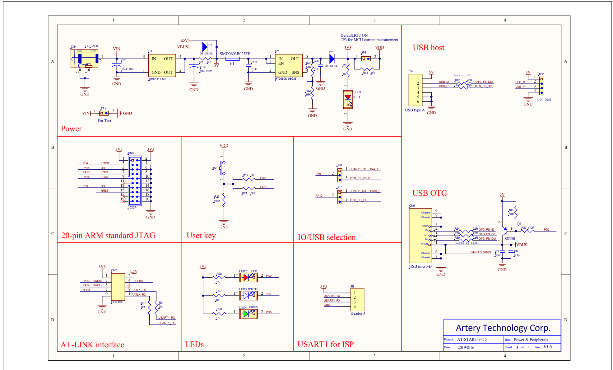
图 8. 原理图(电源和外设)
