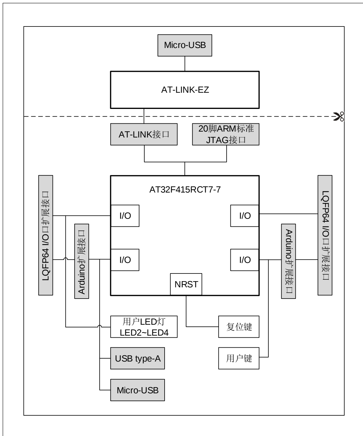
图 2. 硬件框图
