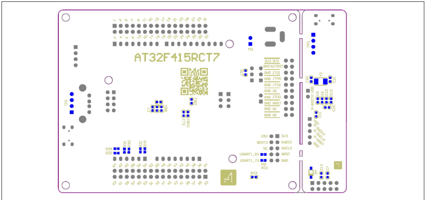
图 4. 底层布局
