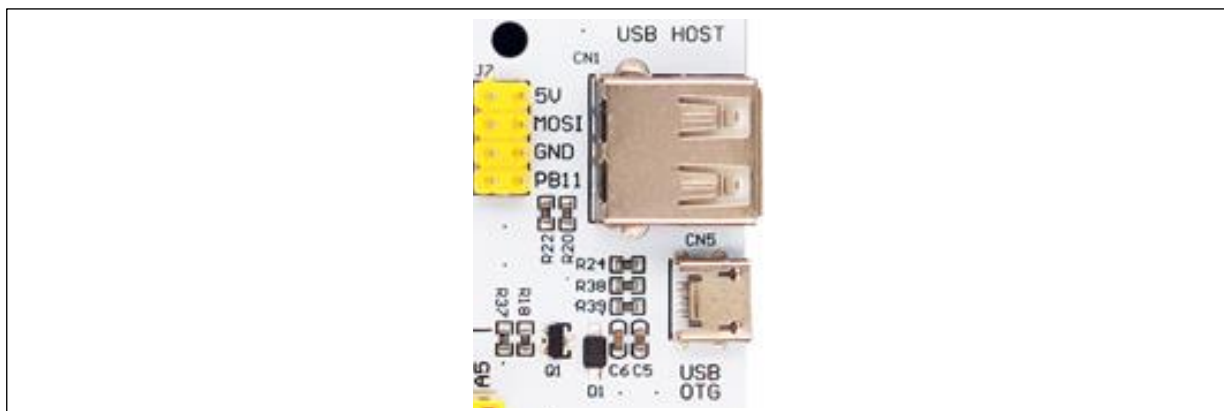
图 5. USB OTG 接口外观
