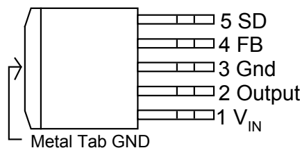
TO263-5L
