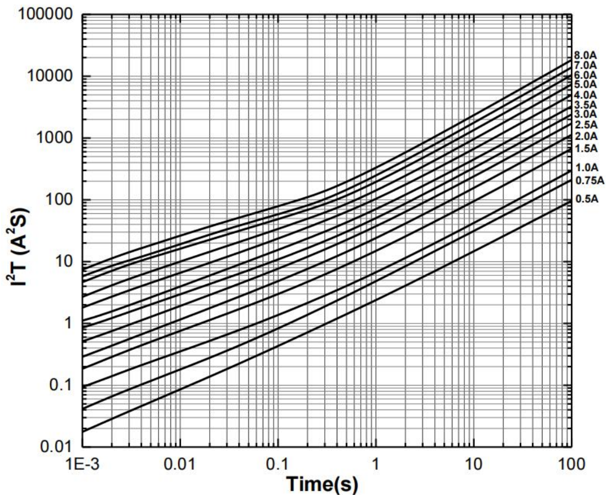
5-3 时间— I^2T 特性曲线/Time- I^2T Curve:
