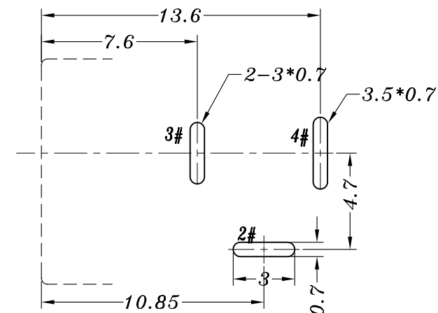
P.C.B LAYOUT
