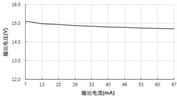
输出电压Vs输出电流(Vin=24V)@B2415LS-1WR3
