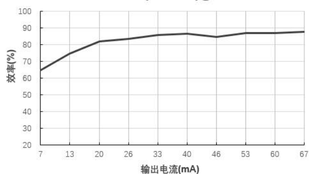
效率Vs输出电流( V_{in}=5V )@B0515LS-1WR3
