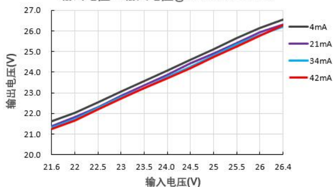
输出电压Vs输入电压@B2424LS-1WR3
