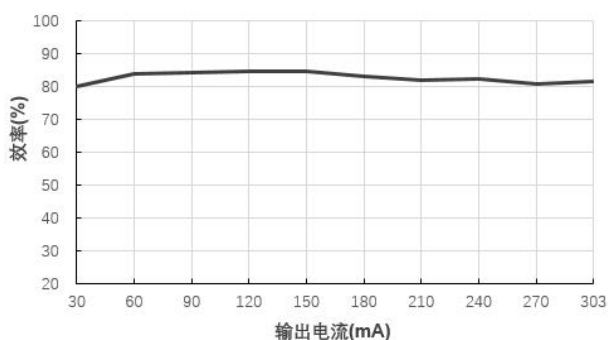
效率Vs输出电流( V_{in}=3.3V )@B0303LS-1WR3
