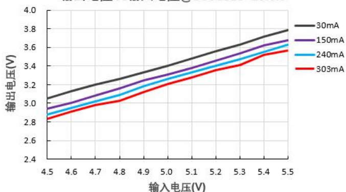
输出电压Vs输入电压@B0503LS-1WR3
