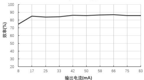
效率Vs输出电流( V_{in}=5V )@B0512LS-1WR3
