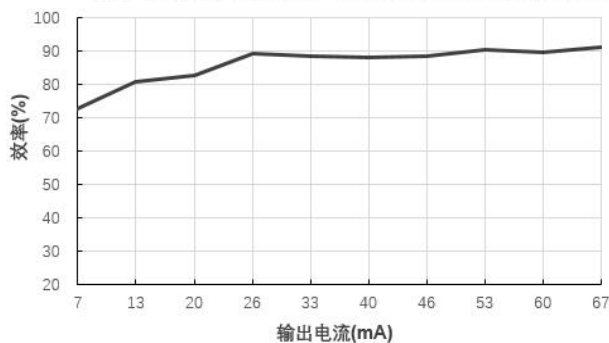
效率Vs输出电流(Vin=24V)@B2415LS-1WR3
