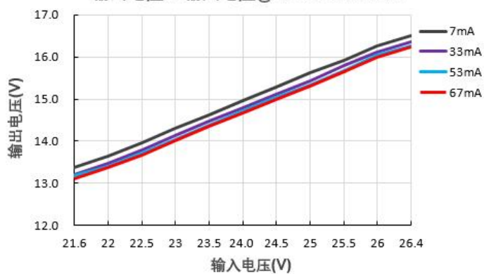
输出电压Vs输入电压@B2415LS-1WR3
