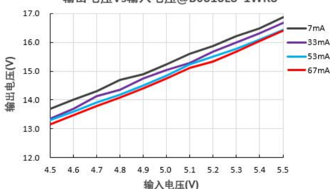
输出电压Vs输入电压@B0515LS-1WR3
