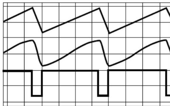
2B 方波占空比-80%
