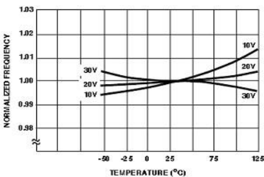
图13. 频率和温度
