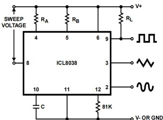
图 5B 频率扫描连接框图
