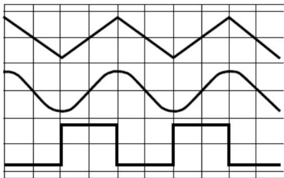
图 2A 方波占空比-50%
