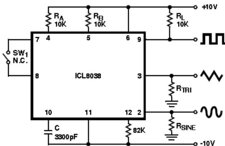
图 1、测试电路
