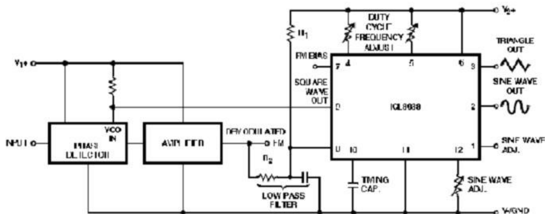
图 9.在相位锁循环电路中, 用作稳呀, 振荡器的波形发生器
