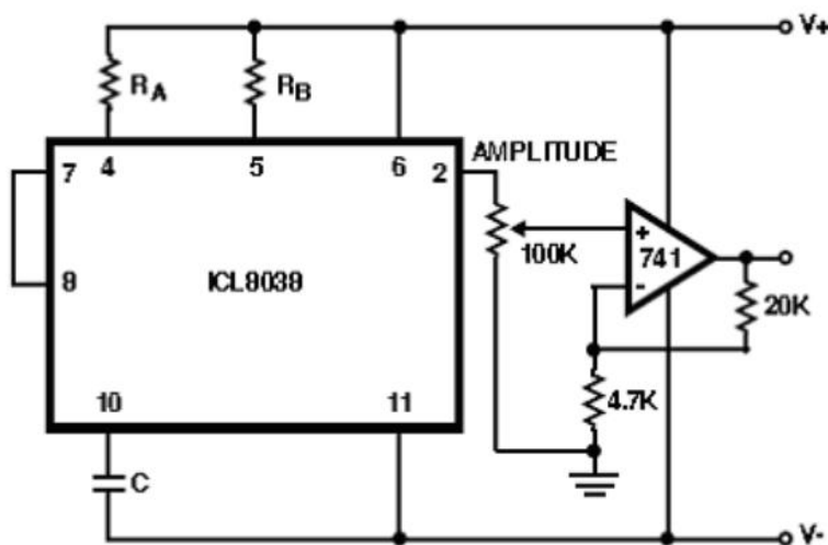
图 6.正弦波输出端缓冲放大器
