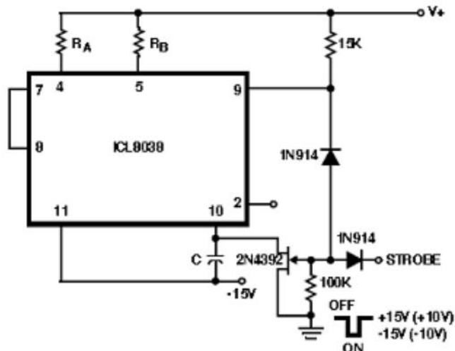
图 7.调制选通发生器
