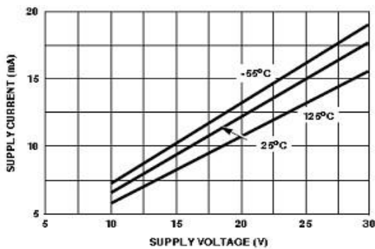
图11. 电源电流和电源电压
