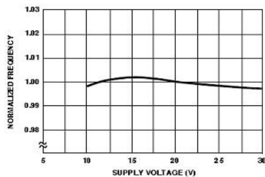
图12. 频率和电源电压
