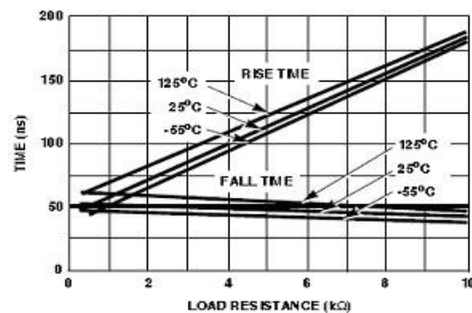
图14. 方波输出端上升/下降沿时间和负载电阻
