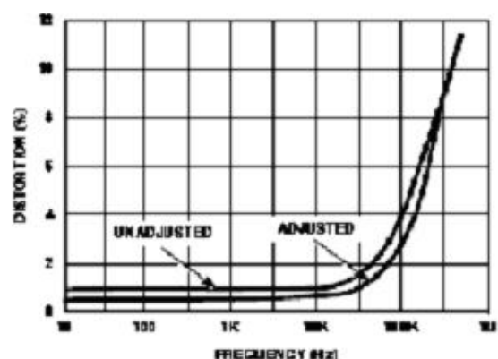
图20.正弦波失调度和频率
