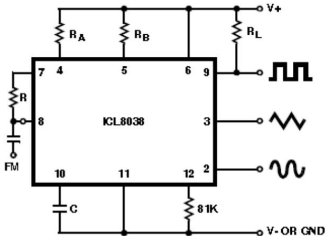
图 5A 频率调制连接框图
