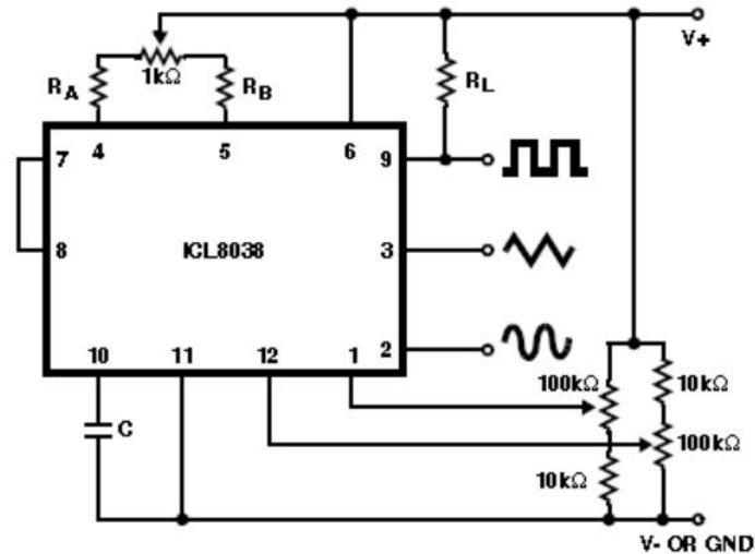
图 4 最小正弦波失真连接框图
