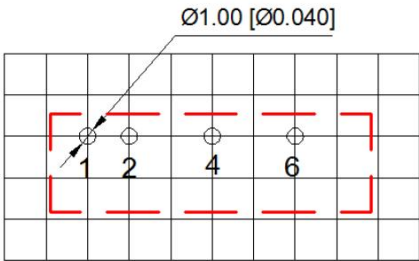
PCB Layout 设计推荐
