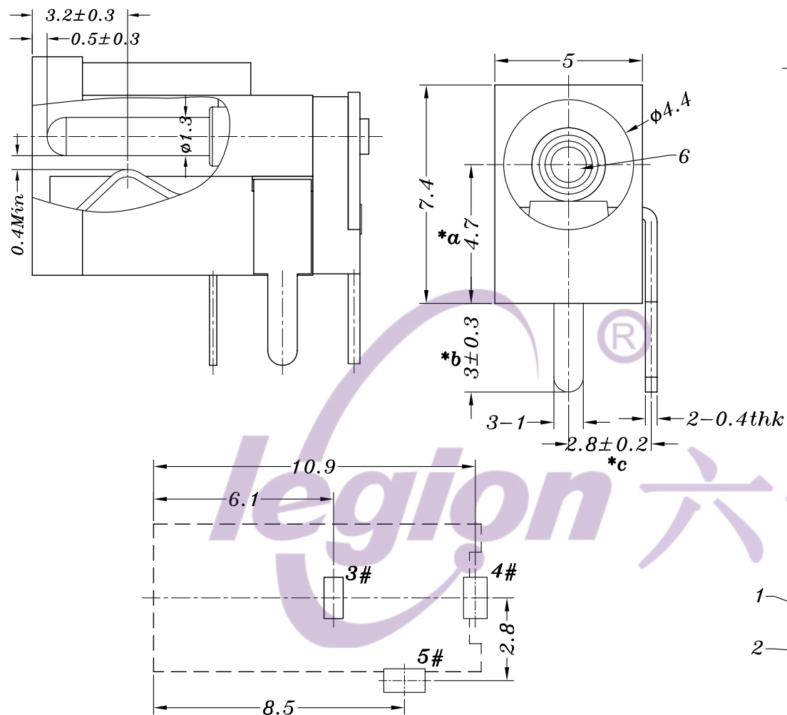
P.C.B LAYOUT
