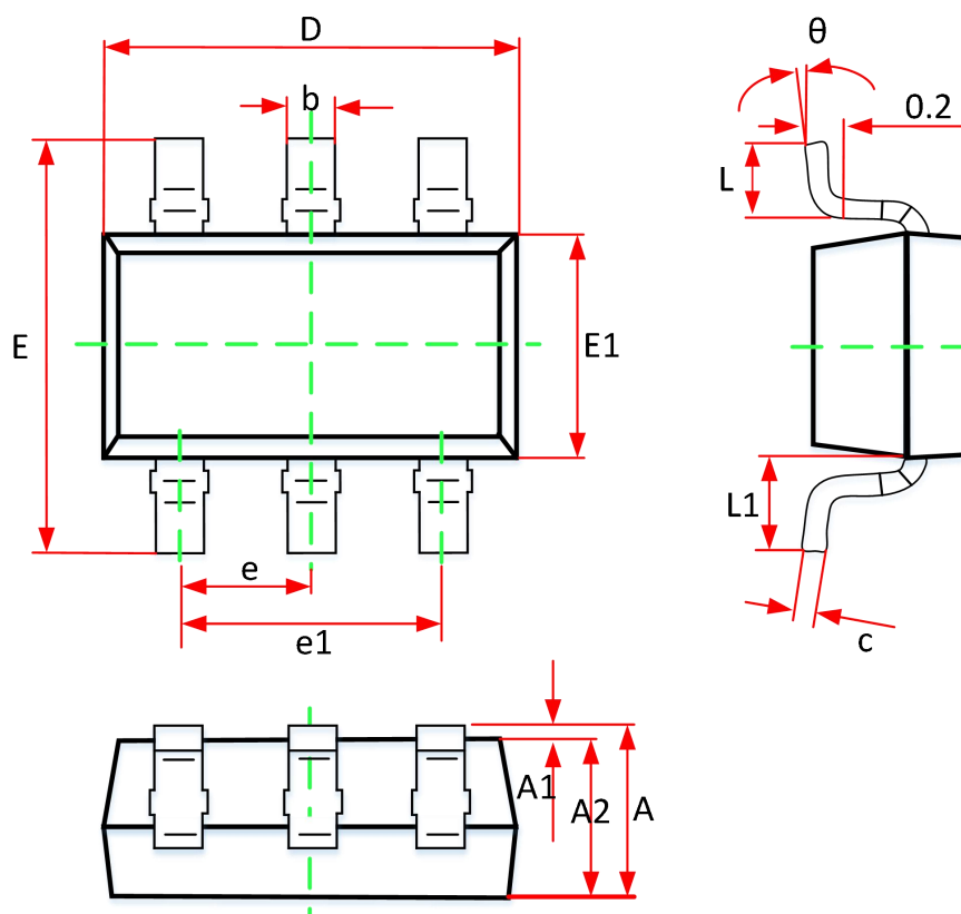
SOT-23-6L 封装信息
