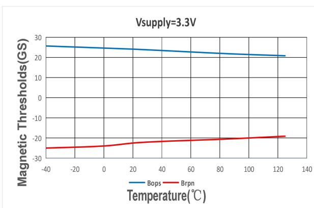
Z 轴磁场阈值 VS 工作温度 @VDD=3.3V
