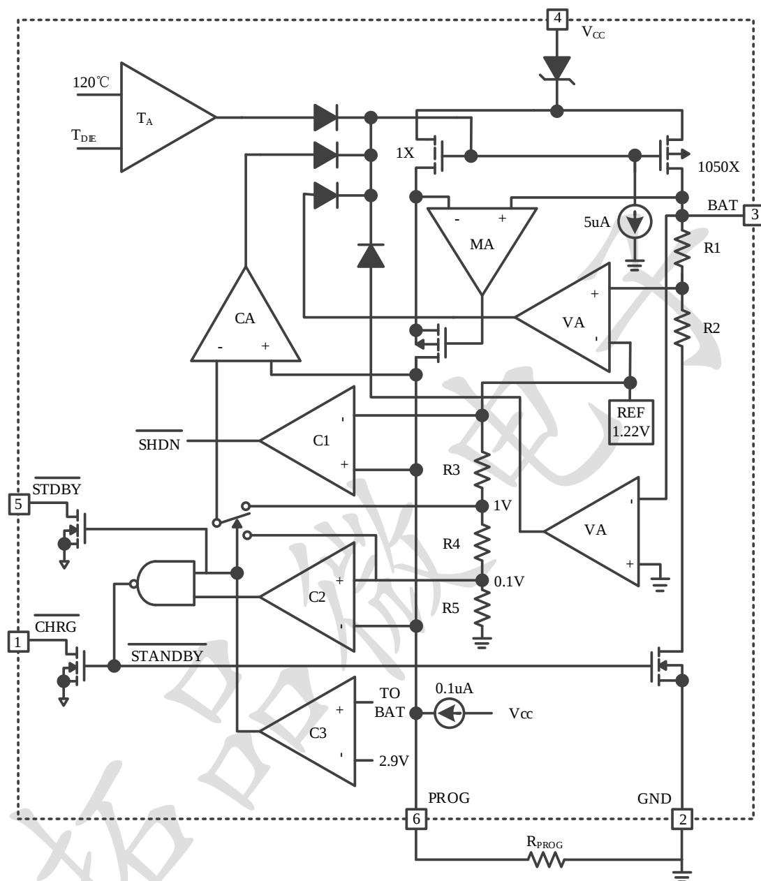
图2 功能方框图
