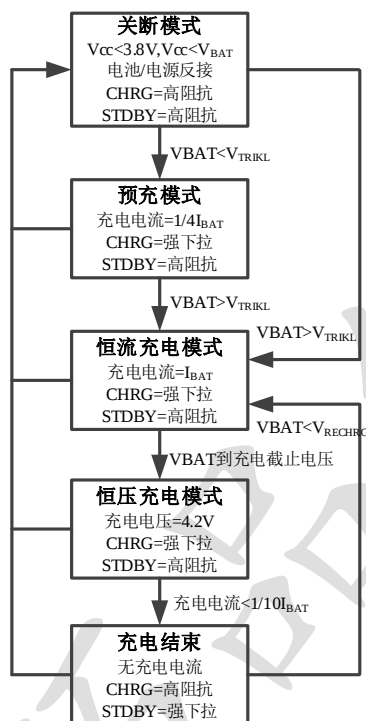
图 3 一个典型充电循环的状态图 电池反接保护功能
