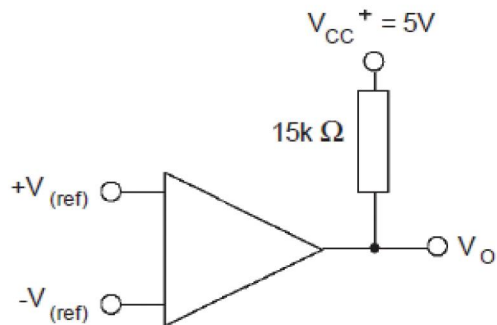
比较器
