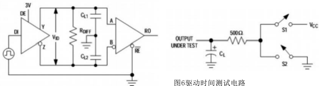
图6驱动时间测试电路
