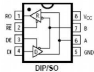
图1封装图
