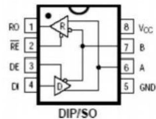
图1封装图
