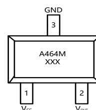
SOT23-3L
