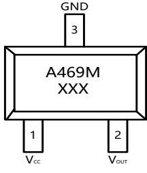
S0T23-3L
