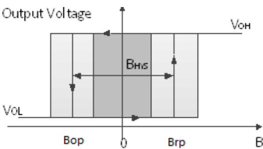
S0T23-3L 输出状态
