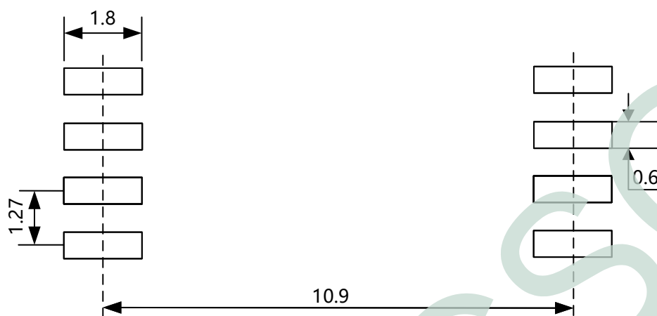
Fig. D1. PCB 焊盘: 8-引脚 SOW
