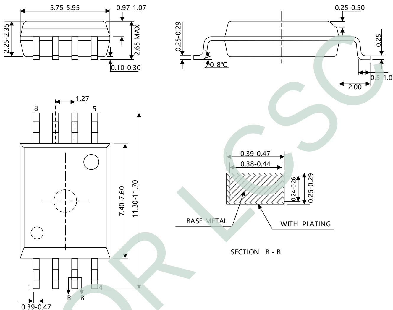
Fig. C1. SOW-8
